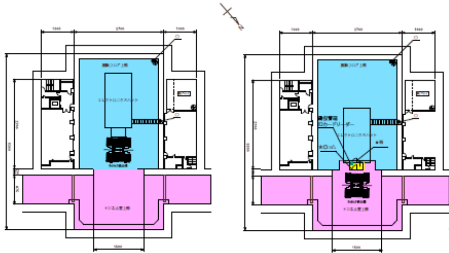
筑波実験棟 B2 Belle2 検出器ロールアウト時 (単位 cm)
