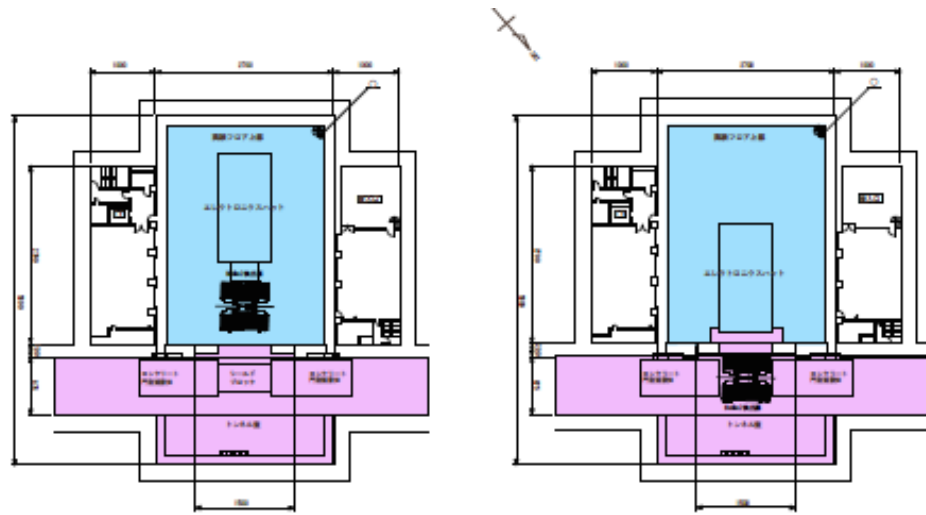
筑波実験棟 B3 Belle2 検出器ロールアウト時 (単位 cm)
