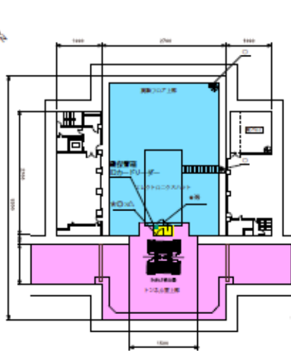
筑波実験棟 B2 Belle2 検出器ロールイン時 (単位 cm)
