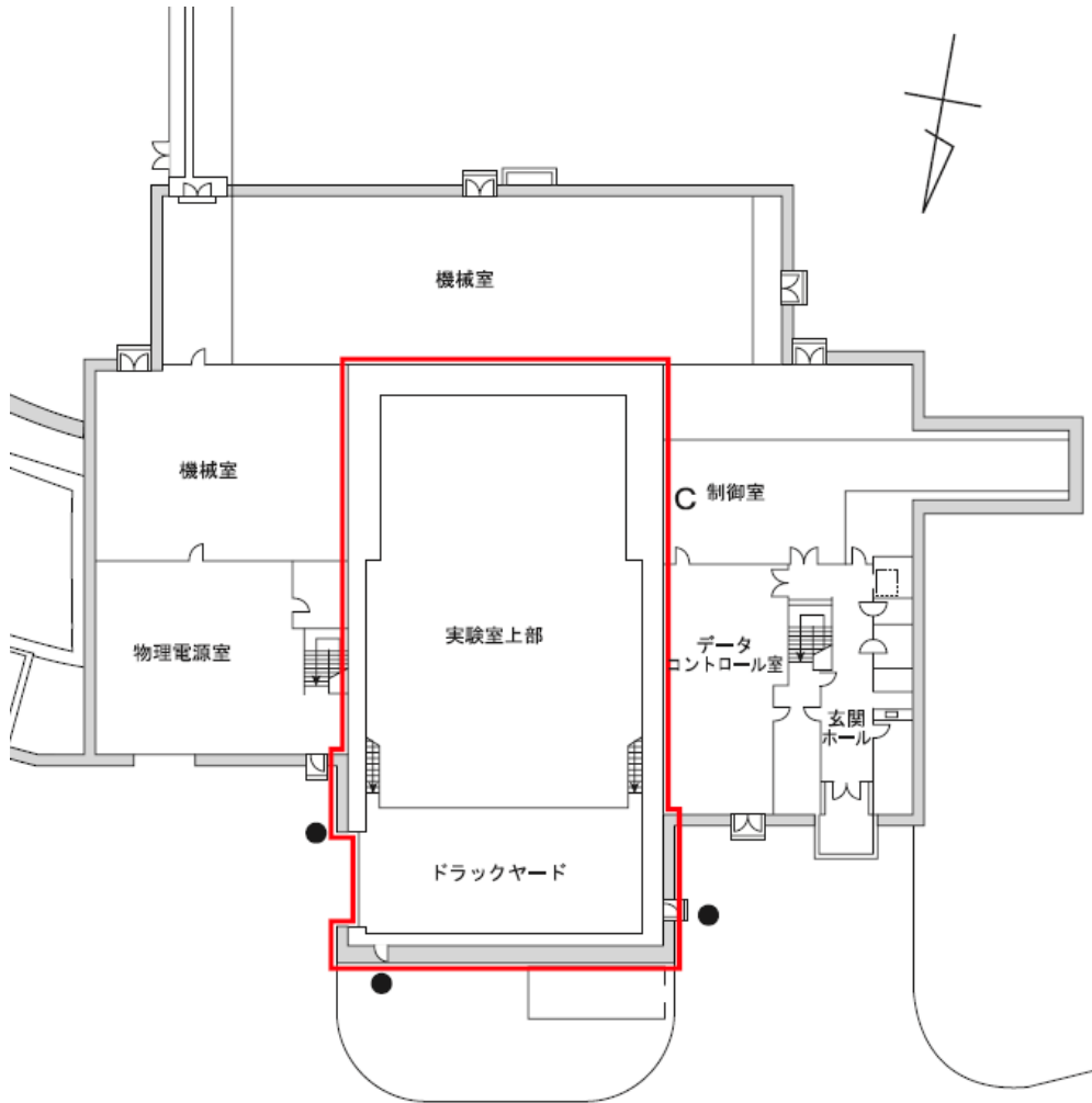
図3 北験準備棟・地上階
