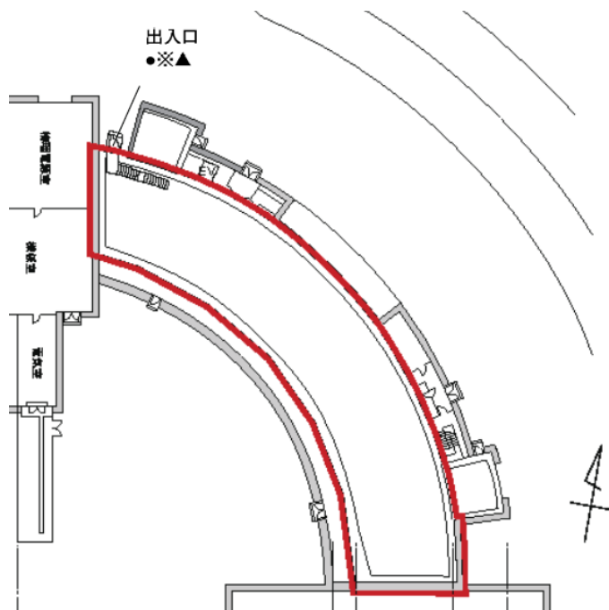
図 6 放射光実験施設・地上階
