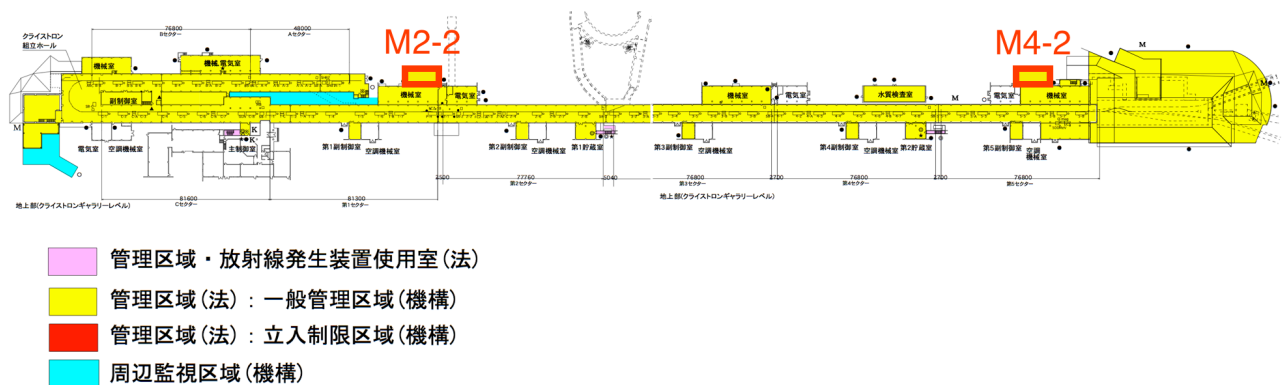
図1 電子陽電子入射器棟地上部の管理区域と該当場所
