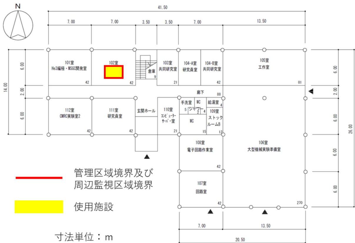
図1 先端計測開発棟（1階）平面図 管理区域及び周辺監視区域（黄色部分）を解除する
