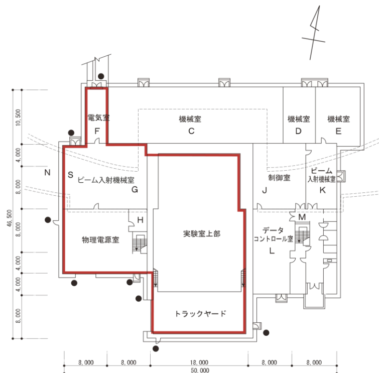
図 1. 南実験棟管理区域変更前
