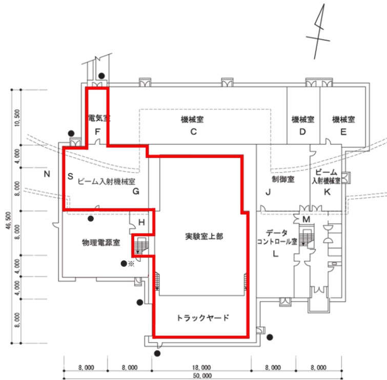
図 2. 南実験棟管理区域変更後(物理電源室が管理区域から一般区域へと変更)
