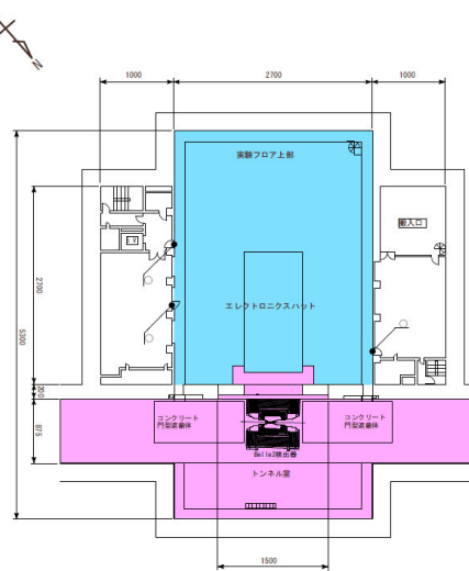
筑波実験棟 B3 Belle2 検出器ロールイン時 (単位 cm)
