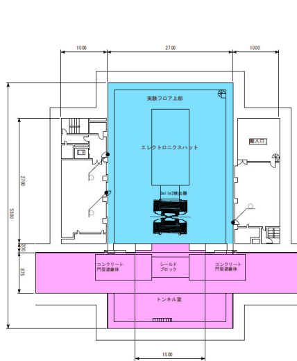
筑波実験棟 B3 Belle2 検出器ロールアウト時 (単位 cm)
