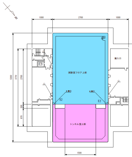
筑波実験棟 B1 平面図 (単位 : cm)
