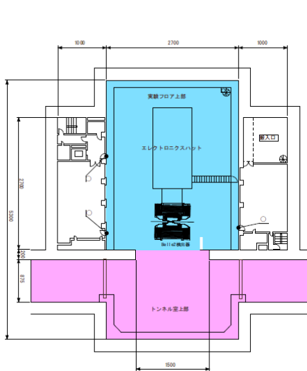
筑波実験棟 B2 Belle2 検出器ロールアウト時 (単位 cm)
