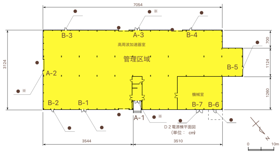
D2 電源棟平面図。全域を放射線管理区域とする（黄色着色部）
