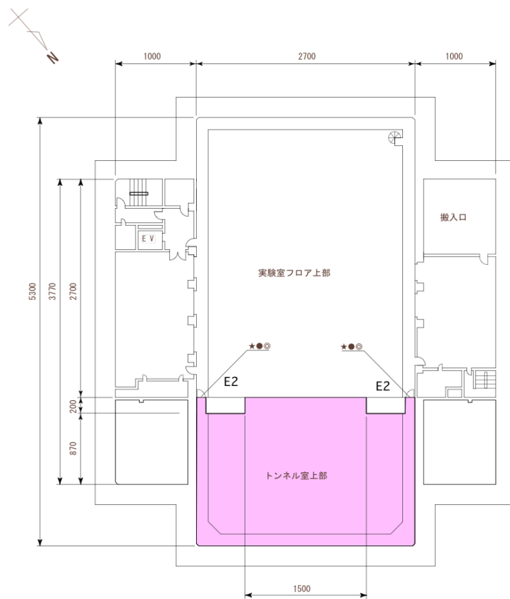
筑波実験棟 B1 平面図 (単位 : cm)
