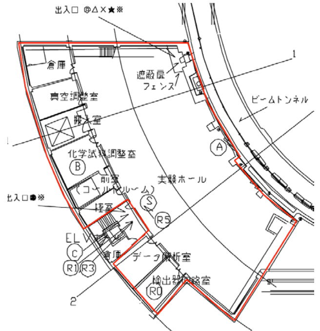
図 2 北西実験棟・地下 1 階
