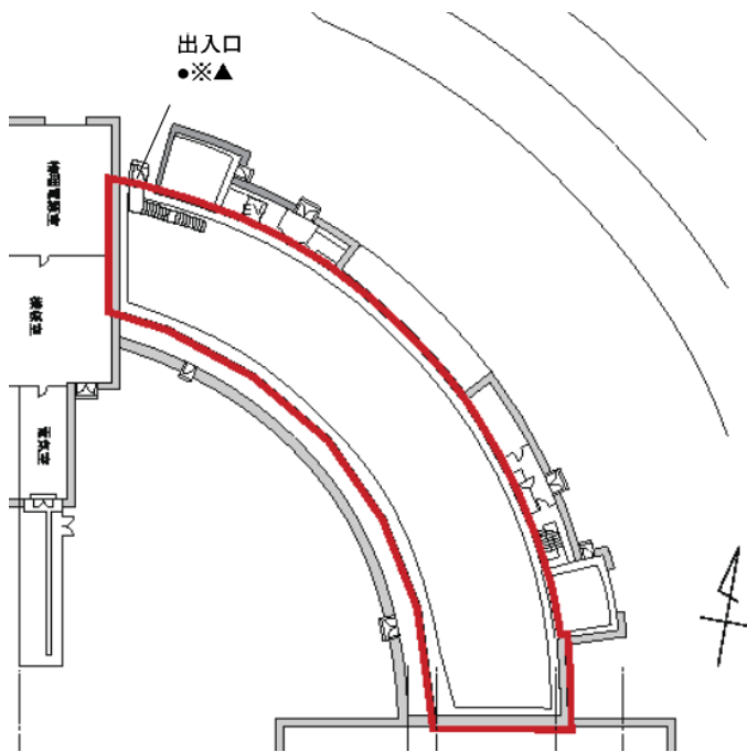
図 6 放射光実験施設・地上階
