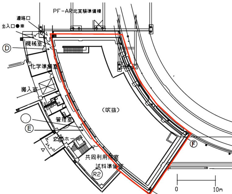
図 1 北西実験棟・地上階
