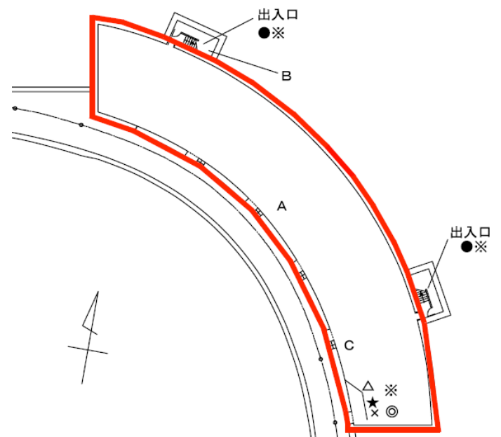
図 7 放射光実験施設・地下 1 階
