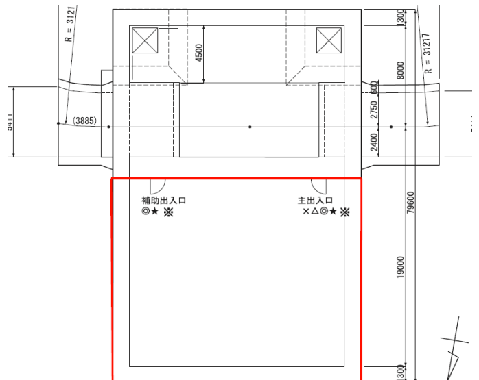
図3 北実験準備棟・地上階
