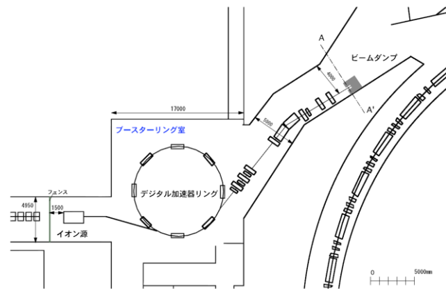
デジタル加速器全体図
