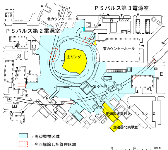
図1 陽子加速器施設(主リング盛土上付近)
