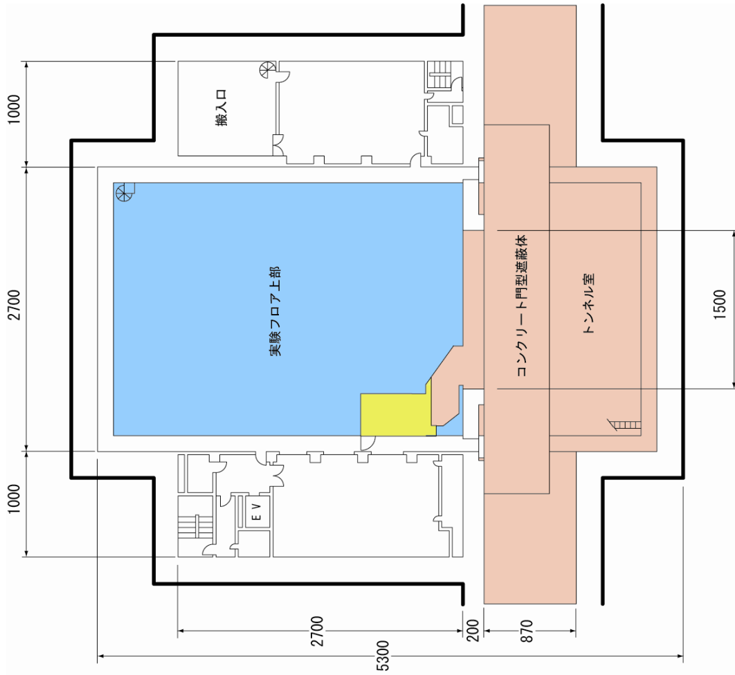
富士実験棟B3平面図 (単位 : cm)
