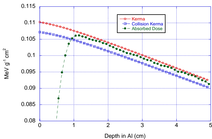
図 2: 6 MeV 光子並行ビームによる Al 体系中のカーマ、衝突カーマ及び吸収線量。
