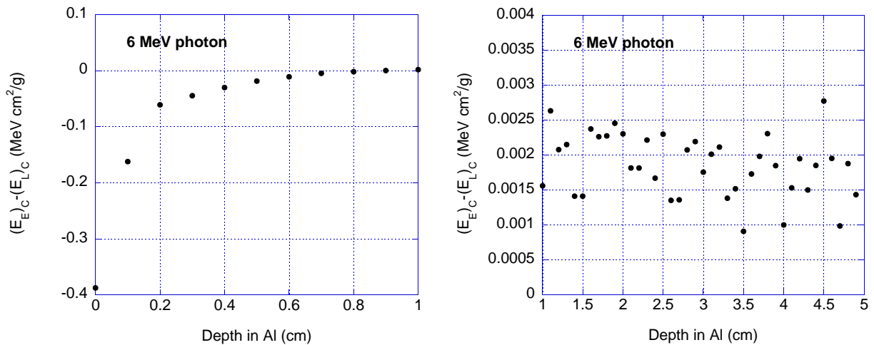
図 3: 1mm の領域への荷電粒子によるエネルギー流入 ((E_E)_C) とエネルギー流出 ((E_L)_C) の差。
