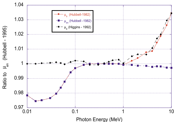
図 1: 公表されているエネルギー移行係数とエネルギー吸収係数の比較例。
