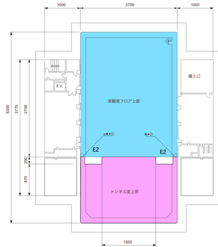
筑波実験棟 B1 平面図 (単位 : cm)
