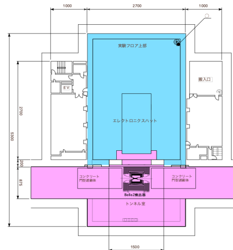
筑波実験棟 B3 Belle2検出器ロールイン時(単位cm)
