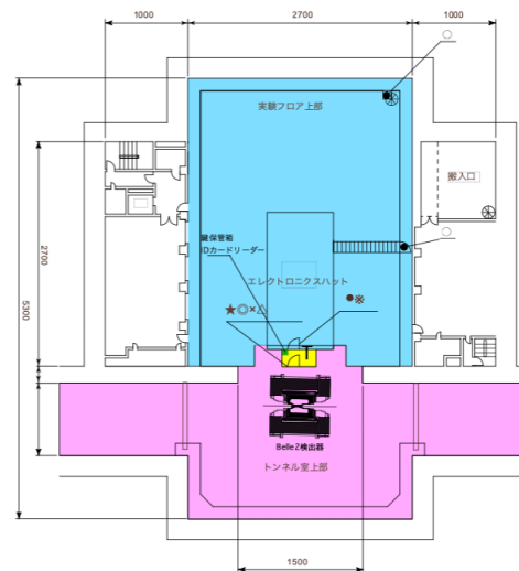
筑波実験棟 B2 Belle2検出器ロールイン時(単位cm)
