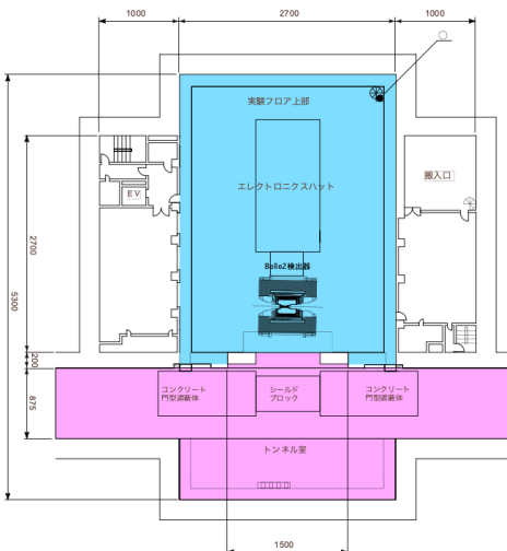
筑波実験棟 B3 Belle2検出器ロールアウト時(単位cm)
