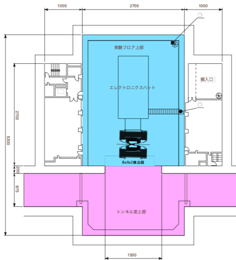
筑波実験棟 B2 Belle2検出器ロールアウト時(単位cm)
