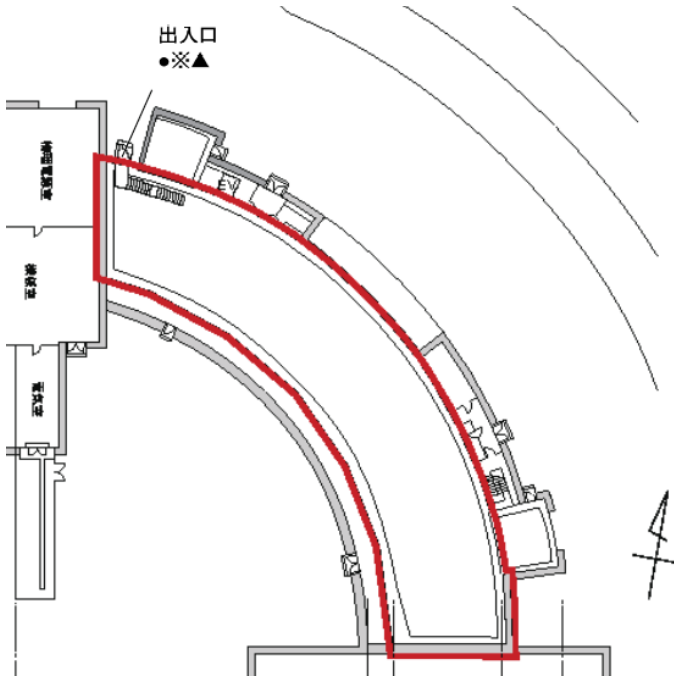
図 6 北東実験棟・地上階
