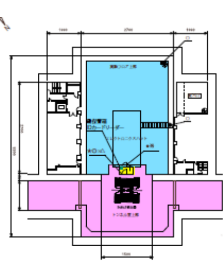
筑波実験棟 B2 Belle2 検出器ロールイン時 (単位 cm)
