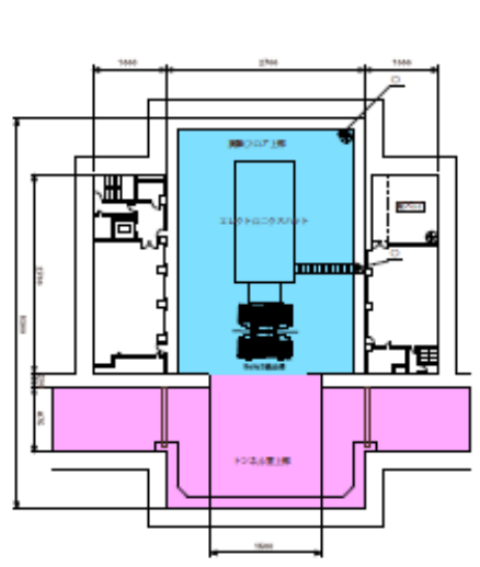
筑波実験棟 B2 Belle2 検出器ロールアウト時 (単位 cm)
