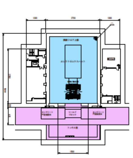
筑波実験棟 B3 Belle2 検出器ロールアウト時 (単位 cm)
