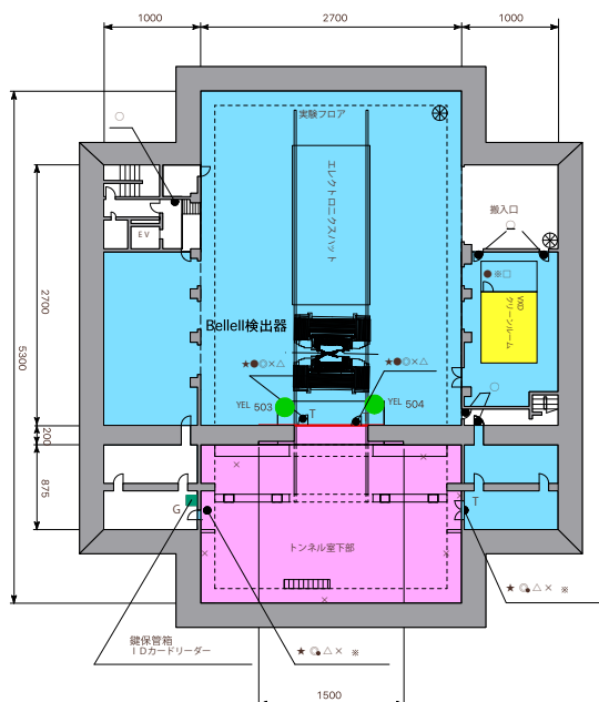
筑波実験棟B Belle 検出器ロールアウト時(単位cm)
