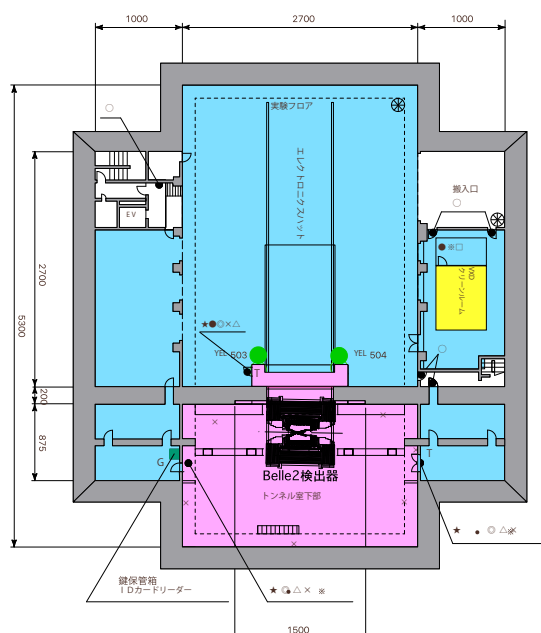
筑波実験棟B Belle 検出器ロールイン時(単位cm)
