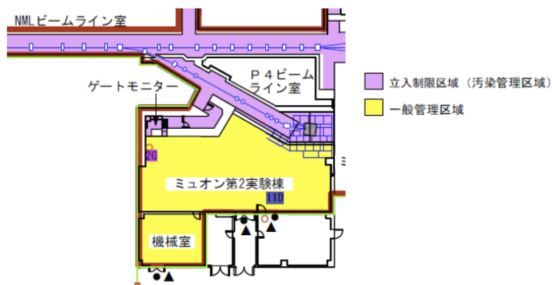
図1：P4 ビームライン室内管理区域（変更前）
