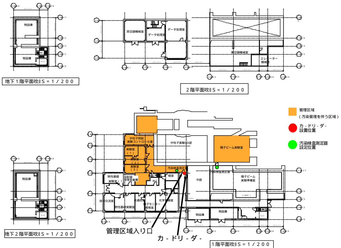
図1：陽子ビーム利用実験棟管理区域(変更後)
