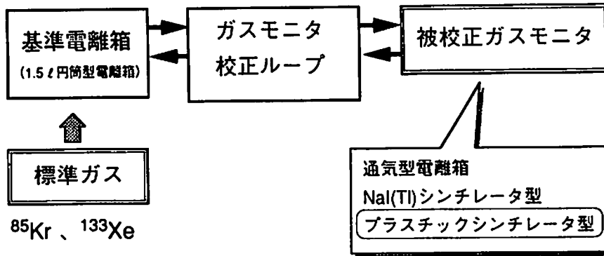
図4 ガスモニタの校正手法
