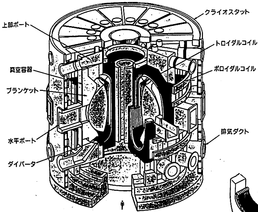
図1 ITER外観
