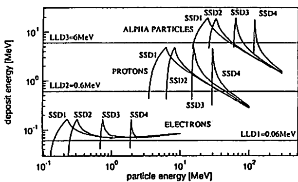
Figure 2. TRIM85(for p, \alpha ), Bethe の式 (for e - ) から求めた入射エネルギーに対する HPM 検出器の SSD 中 に沈着するエネルギー
