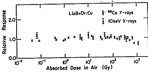
図 8 ^{60}\text{Co} \gamma 線、10 keV X 線に対する \text{Li}_2\text{B}_4\text{O}_7:\text{Cu} の線量特性測定値
