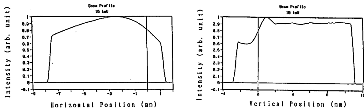
図2 10 keV X線ビーム内プロファイル
