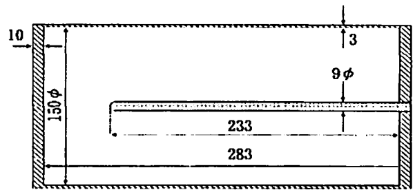
アロカ、トリチウム・モニター MGR-120X 電離箱構造図
