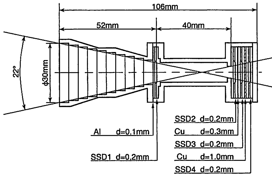
Fig. 1. HPM 検出器断面図 (図中左側が視野方向)
