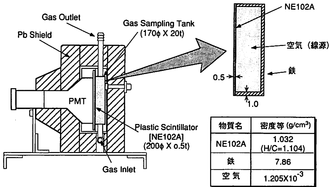
図1 ガスモニタ断面図
