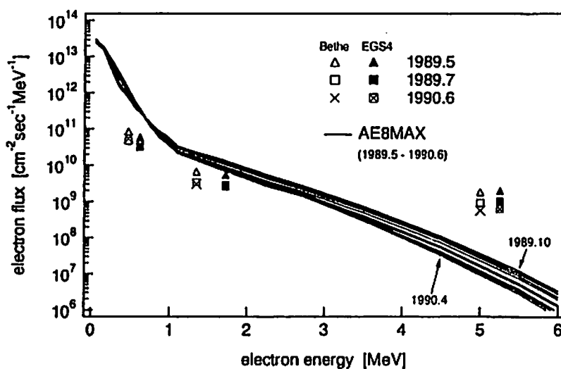
Figure 6. 「あけぼの」による測定値とNASAの電子放射線帯モデル(AE8MAX)から計算した電子エネルギースペクトル
