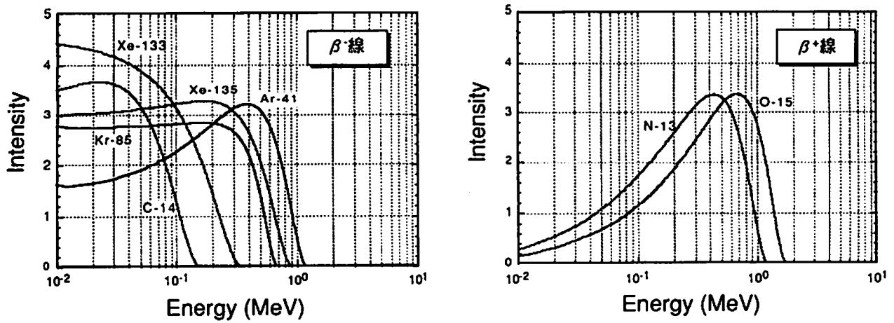
図3 β ± 線エネルギースペクトル
