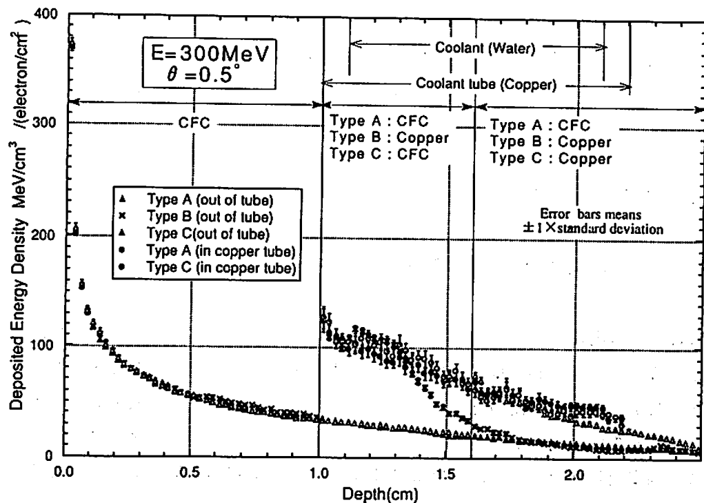
図7 3種類のITER候補ダイバータ断面の平均エネルギー沈着量分布 (逃走電子エネルギー：300MeV、入射角度：0.5°)
