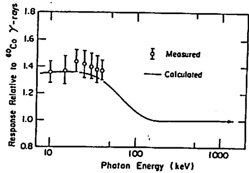
図5 空気中でのLiFレスポンス
