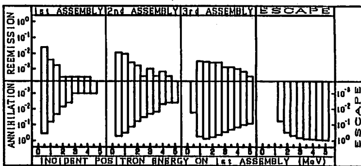
【図2】コンバータから種々のエネルギーの陽電子が入射した場合の多チャンネルモデレータアセンブリーにおける低速陽電子再放出、消滅、透過の確率（計算値）。W表面における再放出分岐率は1/3とした。アセンブリー構成は、第1が2 μm厚W×20枚、第2が2 μm厚W×18枚を2.5 μm厚W2枚ではさんだもの、第3が2.5 μm厚W×20枚とした。
