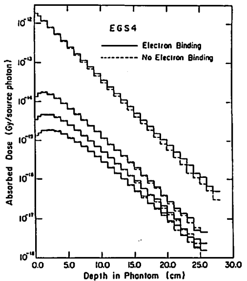
図 1 6 電子束縛の有無による30 keV X線入射時のファントム内吸収線量分布計算値 (EGS4) (6.4 mm 四方ビーム)
