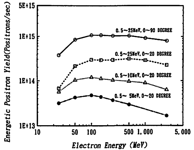
【図5】Taコンバータへの入射電子ビーム（径5mm）の出力を一定（100kW）とした場合の、電子ビームエネルギーとコンバータ（半径5mm以内）からの放出陽電子数との関係（計算値）。図中の数値は放出陽電子のエネルギー及び放出角度範囲。
