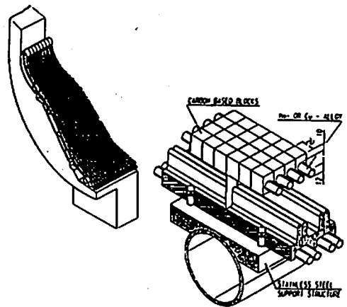
図2 ダイバータ構造例
