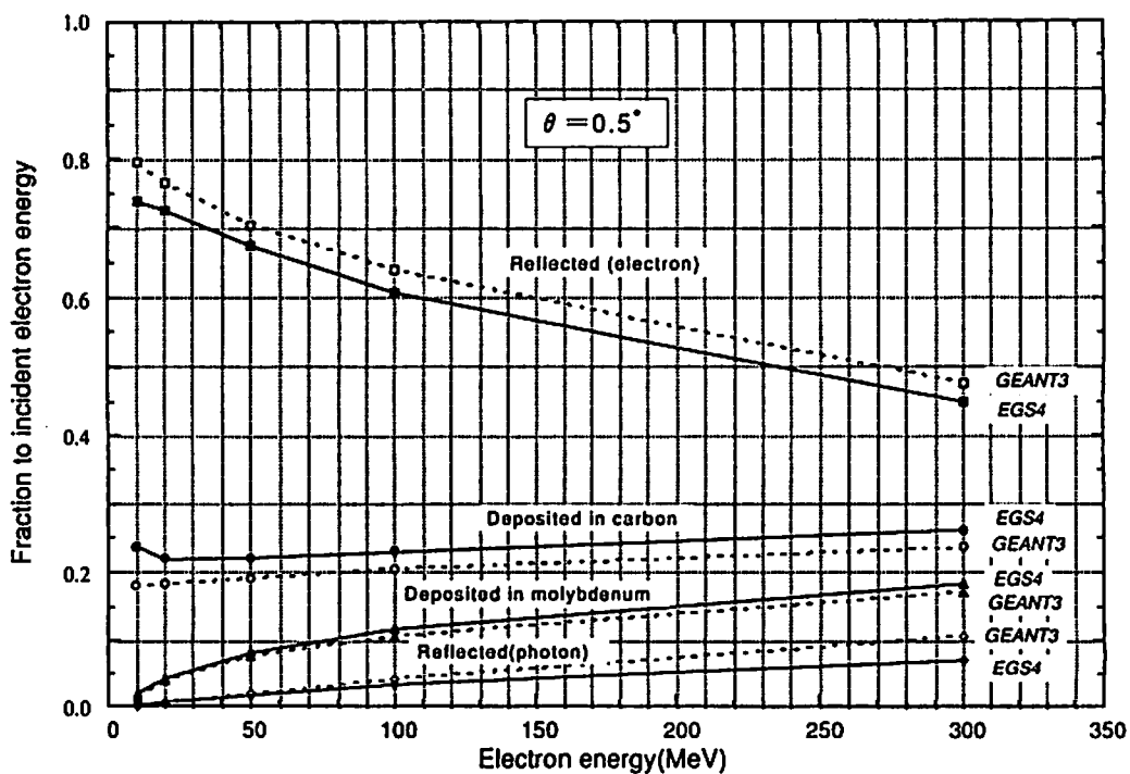
図5 逃走電子の沈着反射割り合い例 (入射角度: 0.5°)
