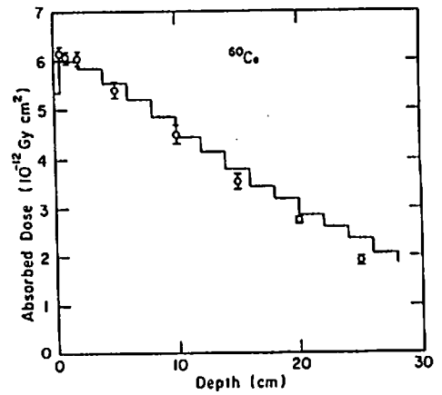
図 11 ^{60}\text{Co} \gamma 線照射時のファントム内吸収線量分布測定値および計算値
