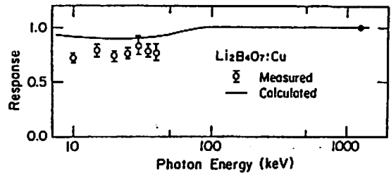
図6 空気中でのLi 2 B 4 O 7 :Cuレスポンス
