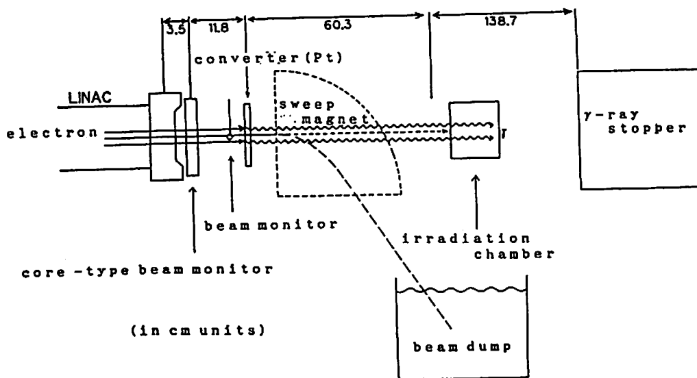
図 1: 照射配置図
