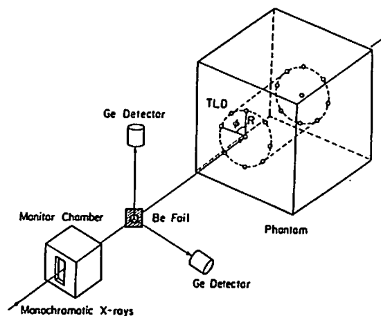
図1 実験配置図
